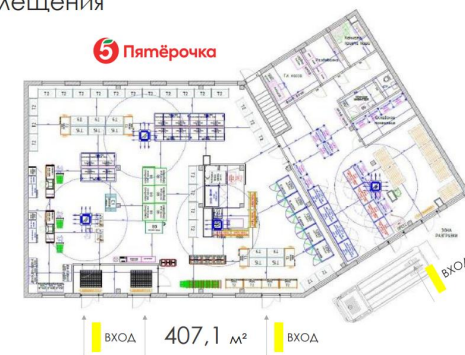
План помещения
