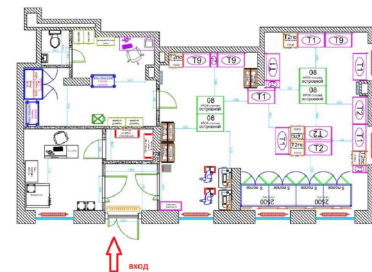
ПЛАН помещения
